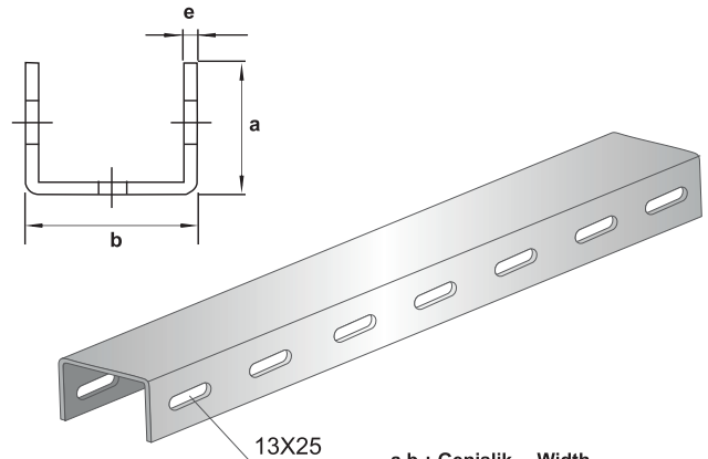
a,b : Genişlik Width h : Yükseklik Height e : Kalınlık Thickness L : Uzunluk Length
